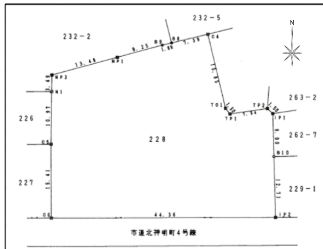
◆ 地積測量図
